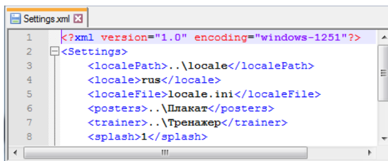
Рисунок 2 – Пример содержимого файла «Settings.xml»
